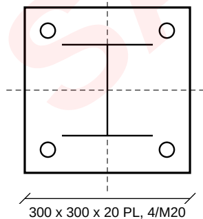
S-101 SCHEDULE: BP1
